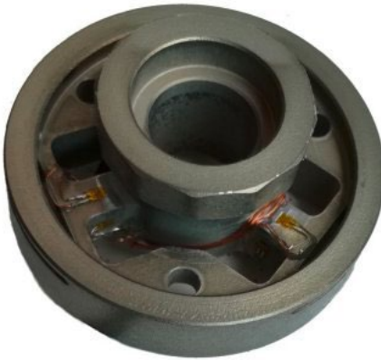
Abb. 17: Blattsensor mit applizierten DMS.
