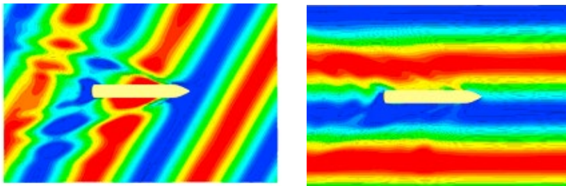
Abb. 5: Berechnete freie Oberflächen-Verformung für Schrägwellen von vorne bei 150° (links) und 90° (rechts)
