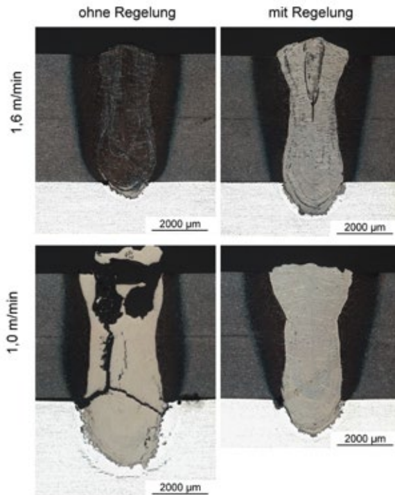
Abb. 10: Querschliffe von Mischverbindungen ohne Einschweißtiefenregelung (links) und mit Einschweißtiefenregelung auf Basis der Kurz-Kohärenzinterferometrie (rechts) bei unterschiedlichen Vorschubgeschwindigkeiten von 1,6 m/min (oben) und 1,0 m/min (unten)
