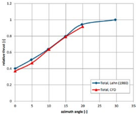
Abb. 2: Vergleich zwischen Messung und Simulation für Thruster-Thruster-Interaktion Einheit der x-Achse.
