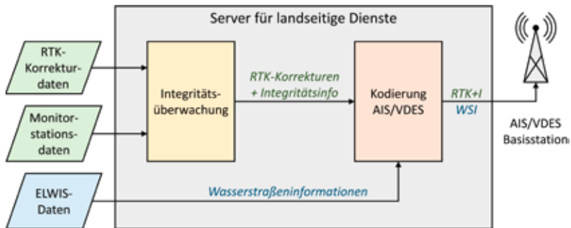
Abb. 2: Detaillierter Systemaufbau des landseitigen Dienstes
