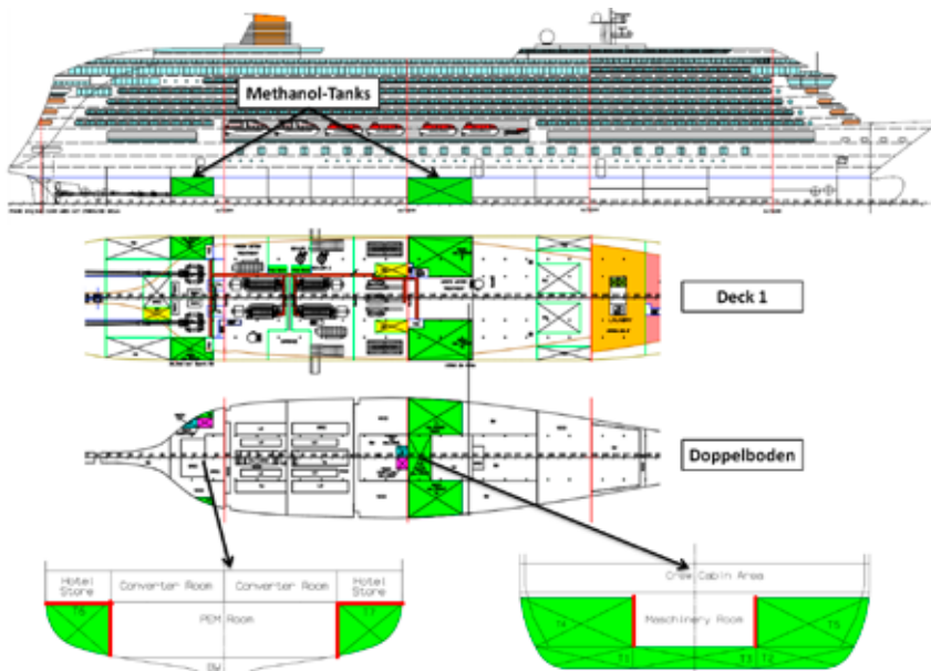
Abb. 5: Methanol-Kreuzfahrtschiff, grün gekennzeichnet sind die Methanol-Lagertanks. Die unteren Schnittbilder verdeutlichen die Positionierung im Doppelboden, an der Seite des Schiffes sowie direkt an der Außenhülle. Dies erlaubt eine optimale Raumnutzung.
