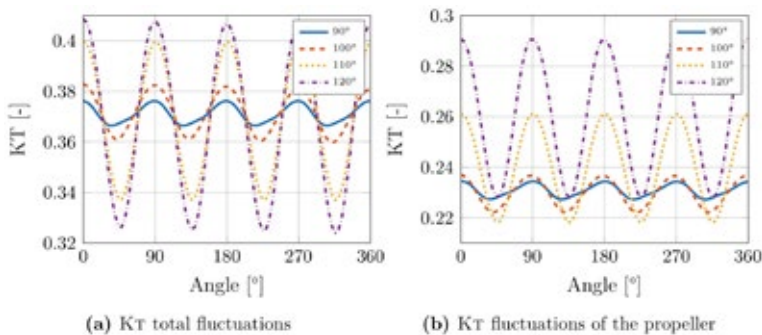
Abb. 5: Spantwinkelvariation, Schubschwankungen während einer Propellerumdrehung
