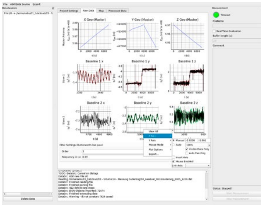
Abb. 6: Echtzeitdarstellung der Rohdaten in der Verwaltungssoftware
