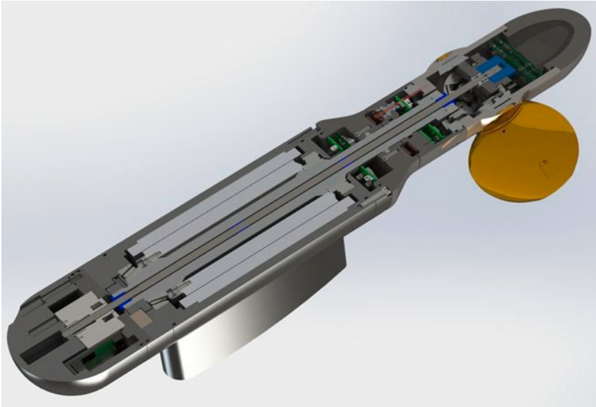
Abb. 14: CPP Schnittbild.
