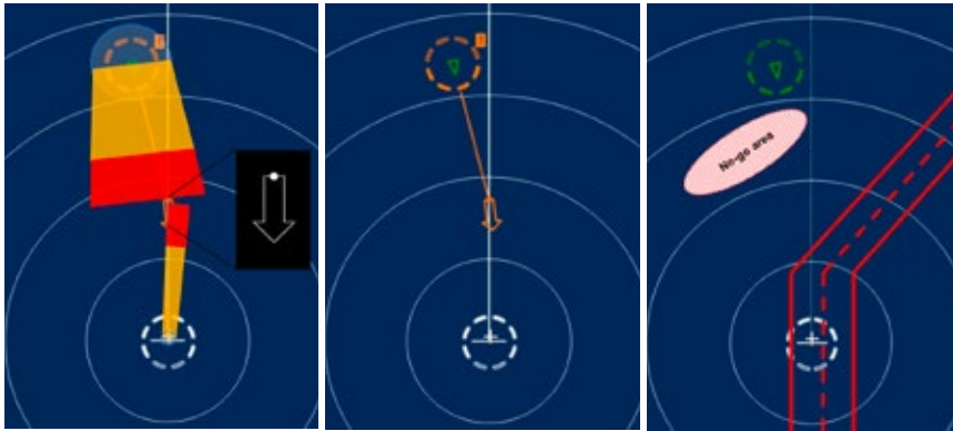
Abb. 5: Die Critical Ship Pose (CSP) zeigt die Pose der nächsten Annäherung auf Basis von Positionsgenauigkeit, Kursschwankung und Geschwindigkeitsschwankung (links mit Visualisierung, mittig ohne Visualisierung). Die CSP wird auf Grund von No-Go-Areas und/oder der Route unterdrückt. Es wird kein Alarm ausgelöst (rechts).
