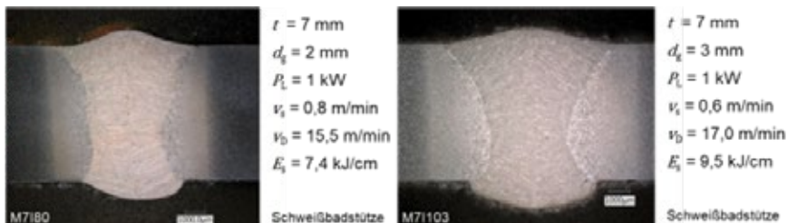
Abb. 2: ShipLight-Prozess am I-Stoß für 7 mm Blechstärke mit einem Spaltmaß von a) 2 mm und b) 3 mm (Quelle: Fraunhofer IAPT)
