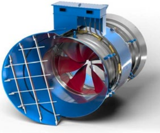
Abb. 1: Aufbau eines Voith Inline Thrusters
