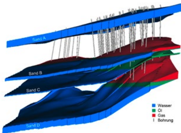
Abb. 18: Das initialisierte Modell (vor Produktionsbeginn) eines Ölfeldes im Golf von Mexiko; 40 Bohrungen, Reservoirfluid-Verteilung [6]
