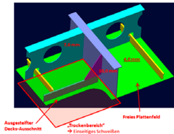
Abb. 12: MEYER WERFT Bauteildemonstrator (Quelle: MEYER WERFT)
