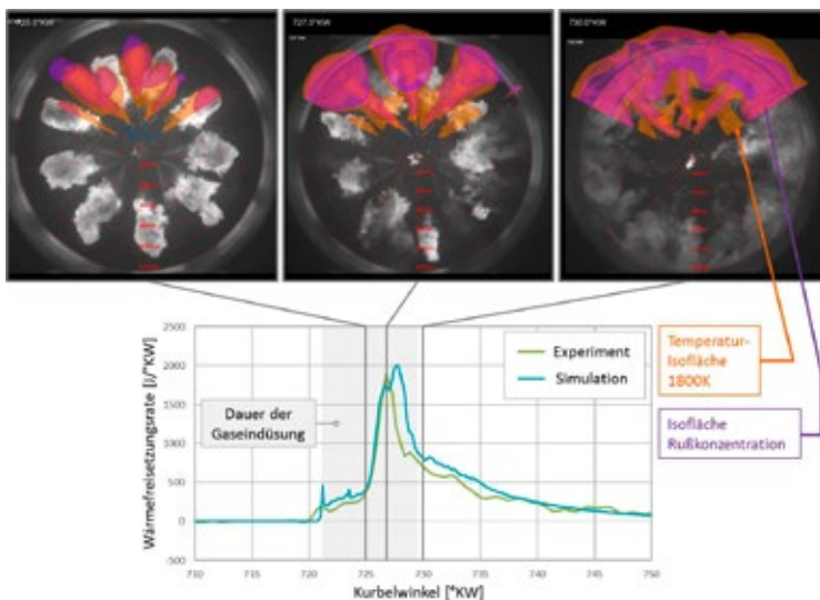
Abb. 9: Am Optikmotor untersuchter HPDF-Betriebspunkt im Vergleich mit der CFD-Simulation
