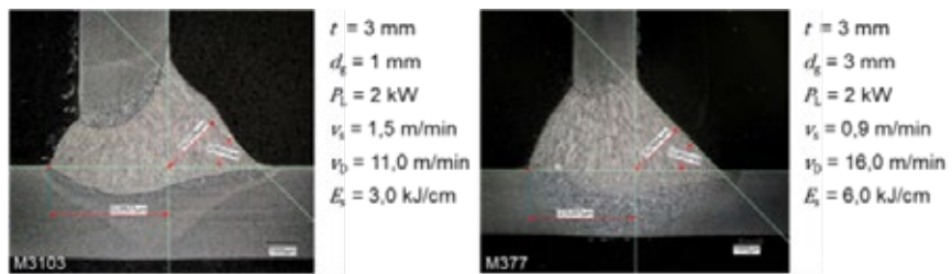
Abbildung 3: Shiplight-Prozess am T-Stoß für 3 mm Blechstärke mit einem Spaltmaß von a) 1 mm und b) 3 mm (Quelle: Fraunhofer IAPT)
