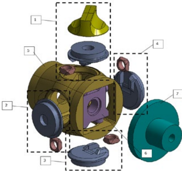
Abb. 21: Komponenten des Verstellmechanismus eines Verstellpropellers.
