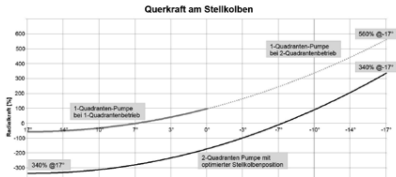
Abb. 4: Querkraft am Stellkolben (Push/Pull-Prinzip)
