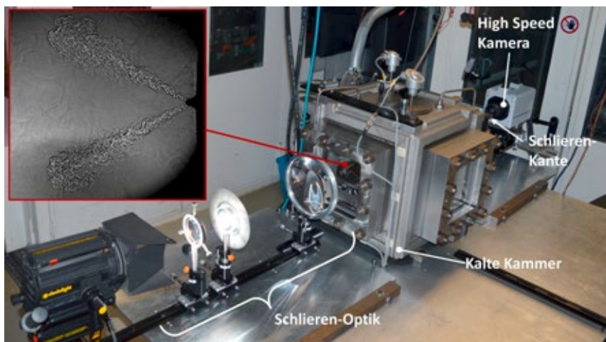
Abb. 6: Schlieren-Bild und -Messaufbau an der Kalten Kammer
