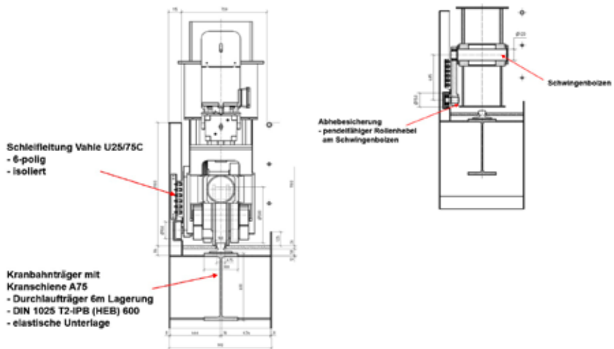
Abb. 7: Entwickelte Lastenleitungsgruppen zur Anbindung des verfahr- und teleskopierbaren Portalkrans an die WATERTRUCK-Schiffsstruktur
