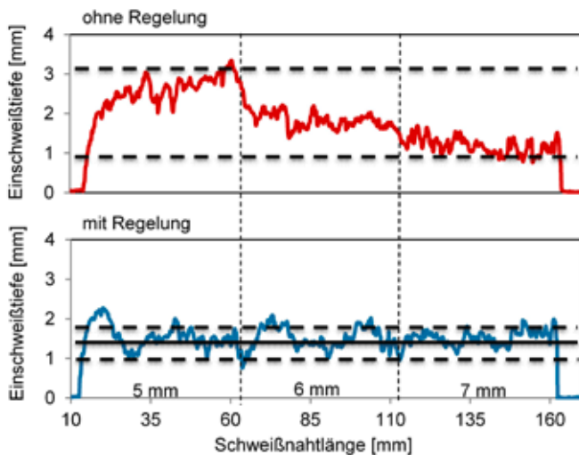
Abb. 12: Einschweißtiefenprofil von Blechdickensprüngen ohne Regelung (oben) und mit Regelung (unten) bei einer Vorschubgeschwindigkeit von 0,8 m/min
