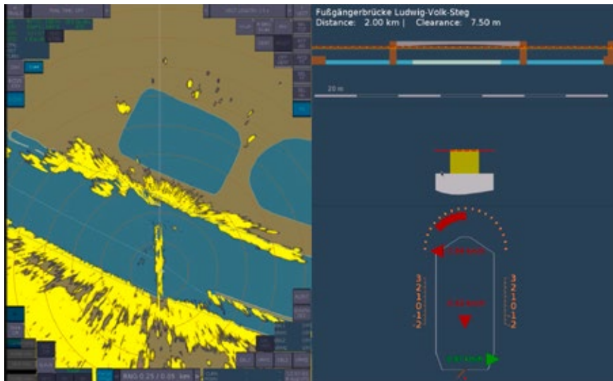
Abb. 15: Conning-Anzeige beim Wenden
