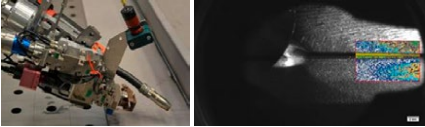
Abbildung 7: a) ShipLight Bearbeitungskopf mit integrierter Fugenfolgesensorik; b) Prozessaufnahme einer Kehlnahtanordnung mit eingblendetem Bereich Region of Interest (ROI) und berechnetem Texturbild (Quelle: Fraunhofer ILT)
