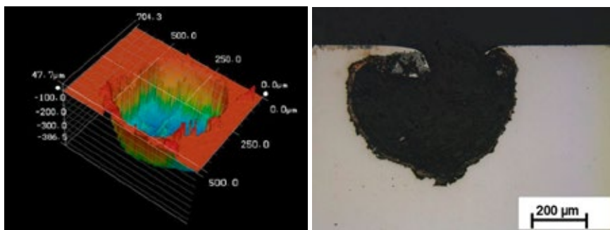
Abb. 30: Korrosionsloch im Stahl 1.4542 nach einer Flächenschädigung von 160 C/cm 2 a) dreidimensionale Darstellung b) Schliffbild
