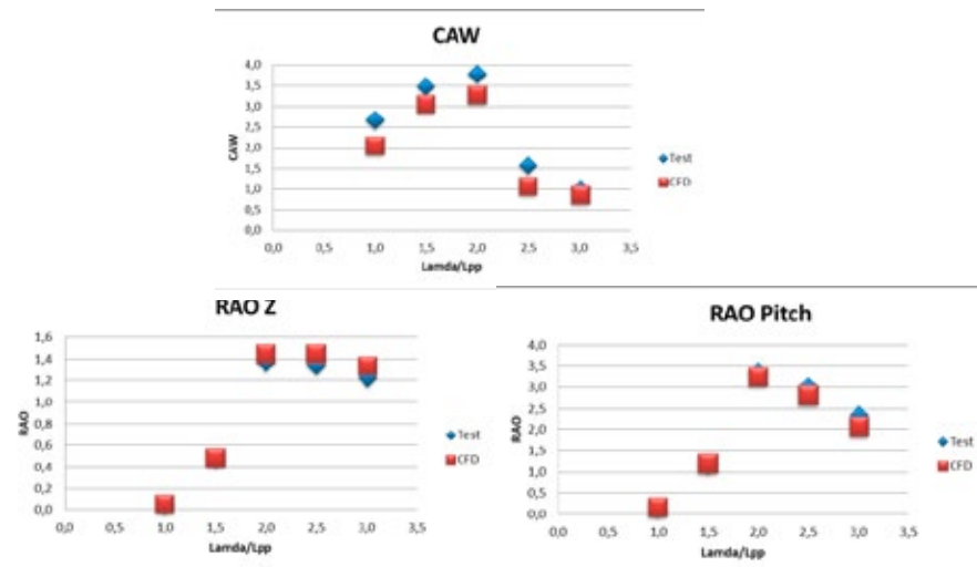
Abb. 8: Vergleich der Zusatzwiderstandsbeiwerte CAW (oben), RAO Tauchen (links) und RAO Stampfen (rechts) zwischen Messungen und CFD-Ergebnisse als Funktion des \lambda/LPP .
