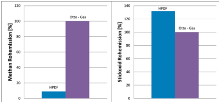
Abb. 10: Relativer Unterschied der Stickoxid Rohemissionen und Methanrohmissionen von HPDF und Gas-Otto Motor
