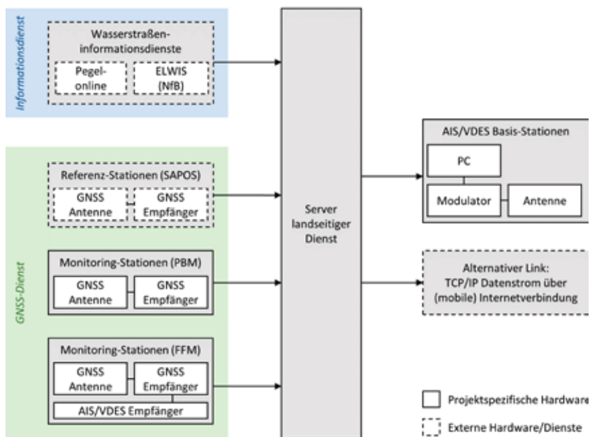
Abb. 5: Landseitige Systemarchitektur
