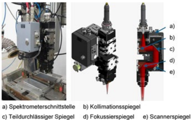
Abb. 3: Versuchsaufbau mit Spanntechnik und Bearbeitungskopf (links) sowie schematische Darstellungen des Bearbeitungskopfes mit optischen Komponenten (mittig und rechts)
