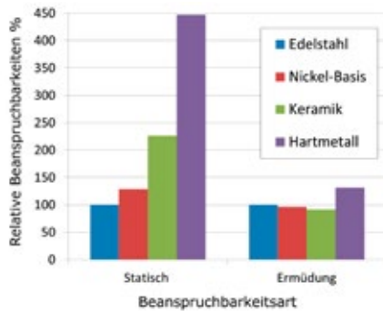
Abb. 23: Experimentell ermittelte Tragfähigkeiten der untersuchten Werkstoffe
