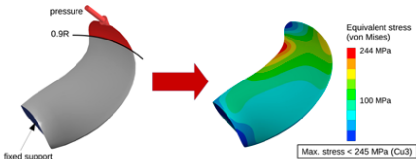
Abb. 8: FEM-Berechnung des Lastfalls 4 der FSICR. Die Eislast wird auf die Druckseite der Propellerspitze aufgebracht. Die automatisierte FEM-Routine bestätigt, dass die maximalen Spannungen nicht überschritten werden.
