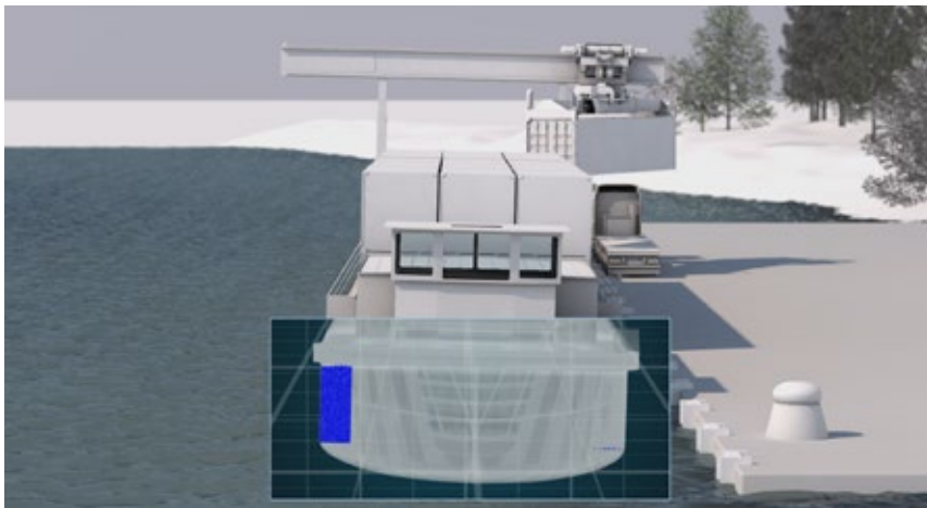
Abb. 11: Mit dem Projekt konzipiertes selbst be- und entladendes Leichtbau-Binnen-Containerschiff
