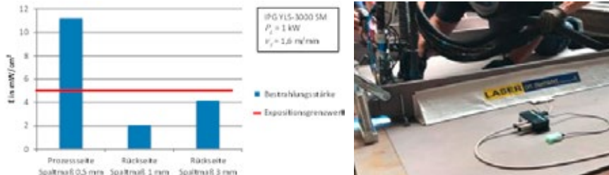
Abbildung 10: a) maximal gemessene Bestrahlungsstärke (Vergleich Prozessseite und Rückseite bei variierenden Spaltmaßen); b) aktive Rückseitenabschirmung (Quelle: LASER on demand)
