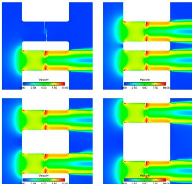
Abb. 2: Geschwindigkeitsverteilung für zwei benachbarte VIT (oben links nur ein VIT aktiv)
