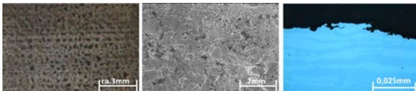
Abb. 29: Anode mit Schäden an den Rohrpositionen 12Uhr a) lichtmikroskopische Aufnahme b) REM-Aufnahme des Schadens c) Schliffbild
