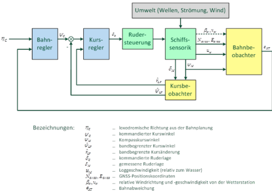
Abb. 9: Kaskadierte Kurs- und Bahnregelung
