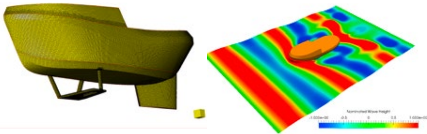
Abb. 7: Oberflächennetz für das VWT (links) und berechnete freie Oberflächen-Verformung für Wellen von vorne bei \lambda/LPP = 1 (rechts).
