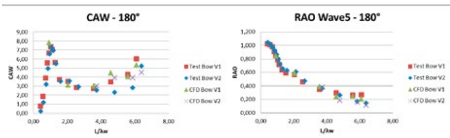
Abb. 6: Vergleich der Zusatzwiderstandsbeiwerte CAW (links), die Übertragungsfunktion (RAO) der Wellen-amplitude hinter dem Schiff (rechts) als Funktion des \lambda/LPP - Verhältnisses zwischen Messungen und CFD-Ergebnissen bei Wellen von vorne.
