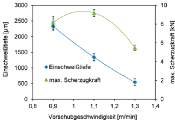
Abb. 5: Max. Scherzugkraft und Einschweißtiefe in Abhängigkeit von der Vorschubgeschwindigkeit
