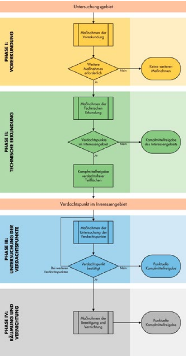
Abb. 2: Phasenschema Offshore-Kampfmittelbeseitigung [6]
