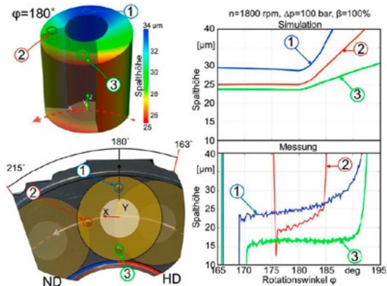
Abb. 14: Vergleich von Messung und Simulation für den inneren Totpunkt (IDC)
