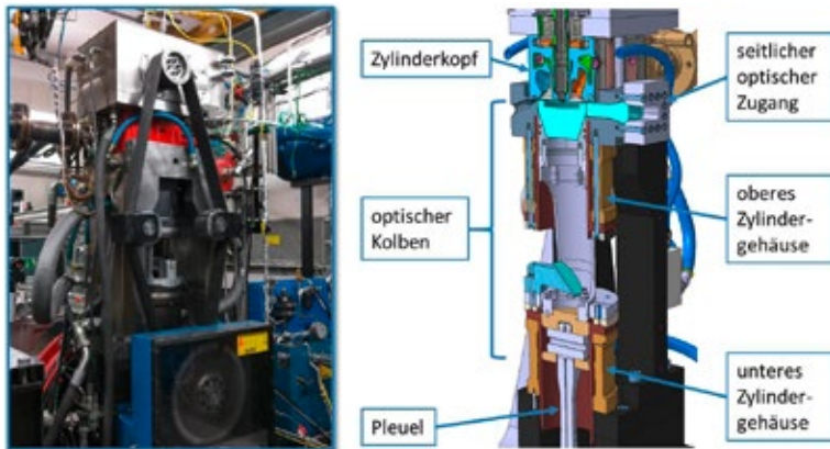
Abb. 8: optisch zugänglicher Einzylinder-Forschungsmotor des LVK
