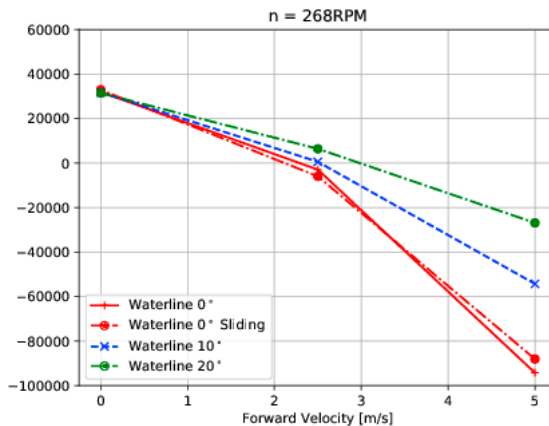
Abb. 12: Querstrahlruder-Schub in Abhängigkeit von der Schiffsgeschwindigkeit und dem Winkel der Wasserlinien am Einbauort. Die durchgezogene Linie zeigt eine aufgelöste Referenzsimulation.
