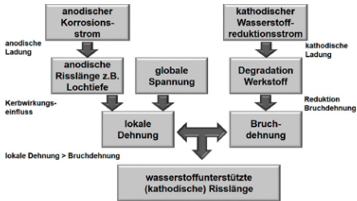
Abb. 28: Schematische Darstellung der Einflussgrößen auf die Risskorrosion nach [15]
