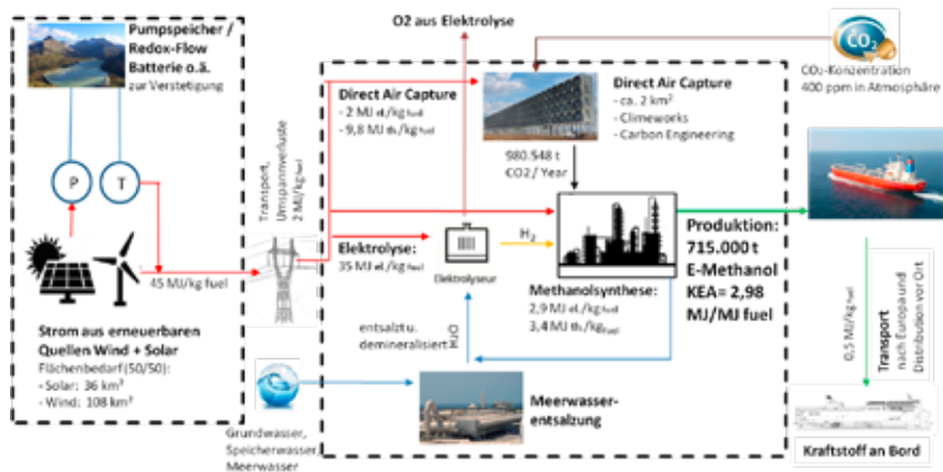
Abb. 12: Schematische Darstellung einer klimaneutralen E-Fuel-Produktionsanlage für Methanol, die \text{CO}_2 als Rohstoff aus der Atmosphäre entnimmt.
