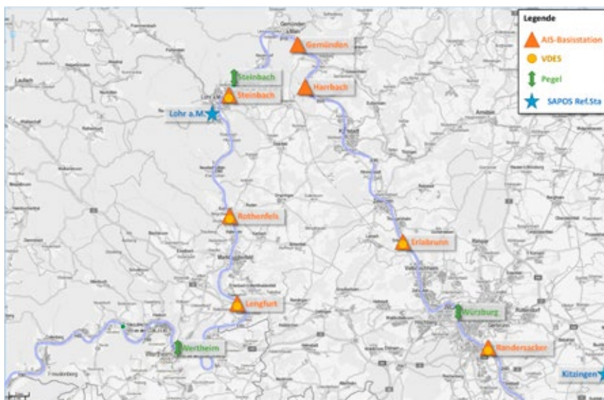
Abb. 3: Aufbereitung der RTK-Korrekturdaten für die AIS-Standorte
