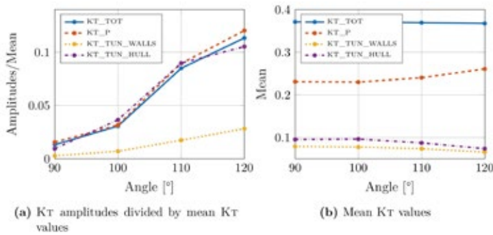
Abb. 4: Spantwinkelvariation, Schubbeiträge, Schubamplituden und Mittelwerte als Schubbeiwert
