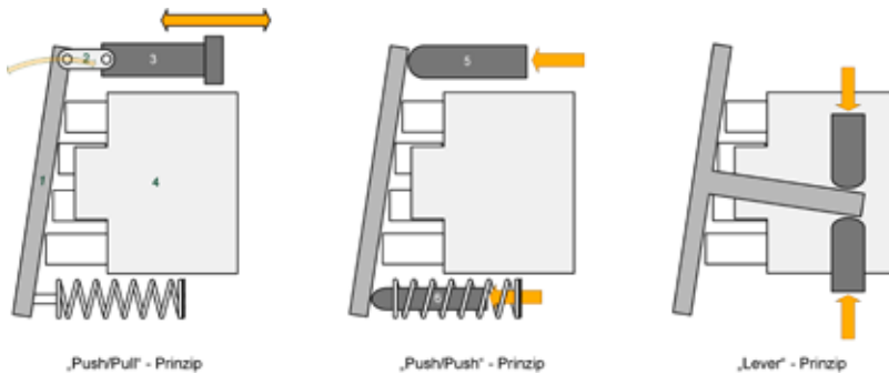
Abb. 3: Vergleich Stellsysteme
