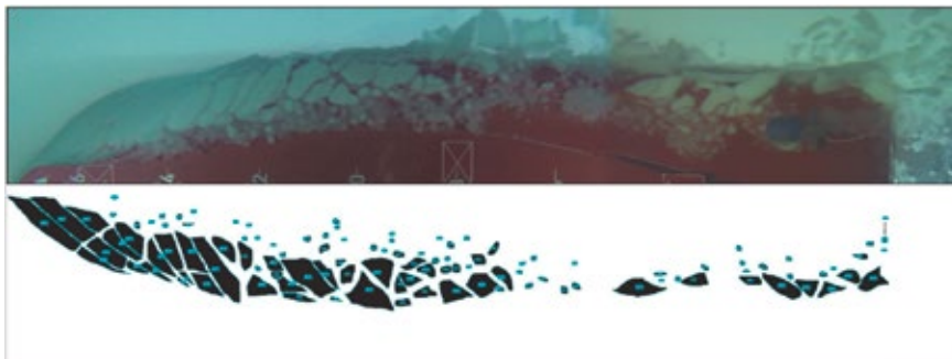
Abb. 7: oben: Unterwasservideoaufnahme des Schollenflusses entlang eines Schiffmodells; unten: identifizierte Schollen nach Anwendung der Bild-Analyse Methodik.
