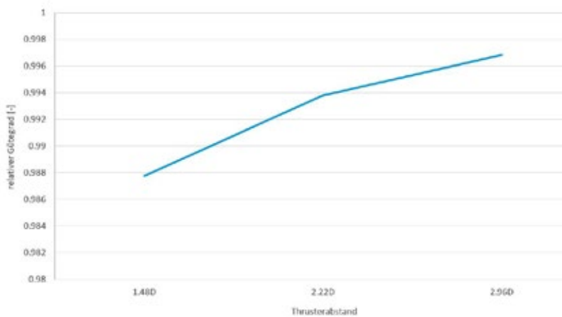
Abb. 3: Prozentualer Gütegradabfall bei Betrieb benachbarter VIT
