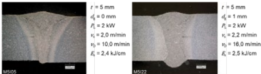
Abb. 1: ShipLight-Prozess am I-Stoß für 5 mm Blechstärke mit a) technischem Nullspalt und b) einem Spaltmaß von 1 mm (Quelle: Fraunhofer IAPT)
