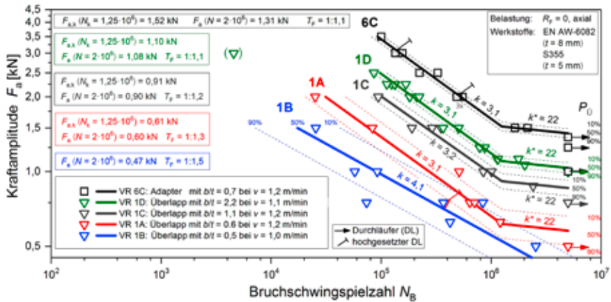
Abb. 8: Schwingfestigkeitsergebnisse für Überlappnähte und Adapter der Variante 1
