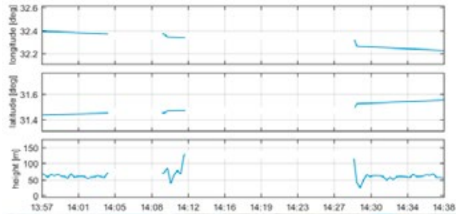
Positionslösung der Empfänger am 12. September
