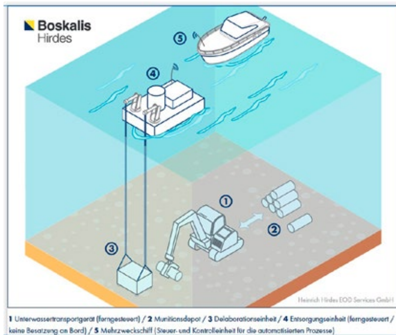
Abb. 1: Offshore-Delaborationsprozess inkl. Technik für großformatige UXO [2]
