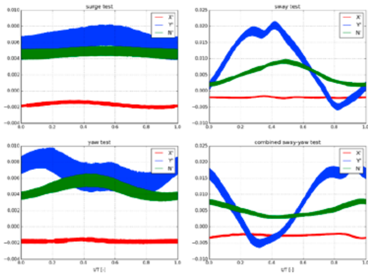
Abb. 8: Berechneter Verlauf der Kräfte und der Momente bei der Bestimmung der Manövrierkoeffizienten
