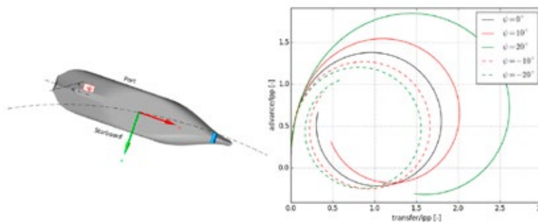
Abb. 10: Berechnetes Drehkreismanöver mit unterschiedlichen Azimuthwinkeln
