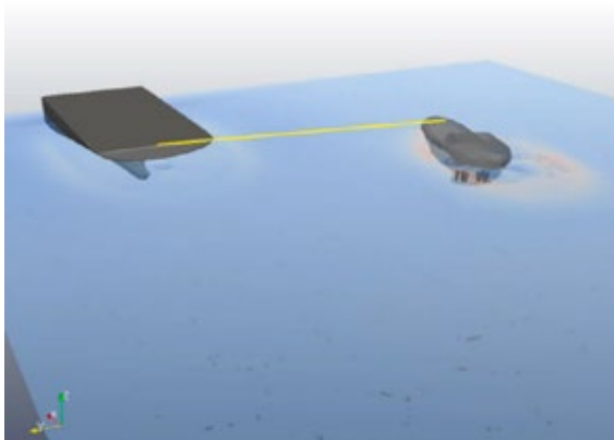
Abb. 13: Simulation der Interaktion von Schlepper und Schiff während eines Escort-Manövers beim indirekten Schleppen.
