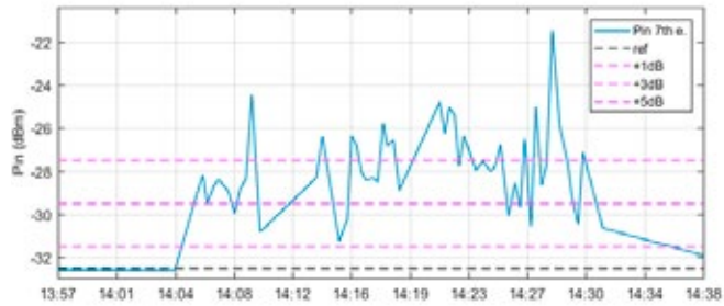
ADC Eingangsleistung Antenne Nr. 7 am 12. September
