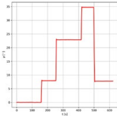
Abb. 7: Ergebnis des statischen Drehversuches
