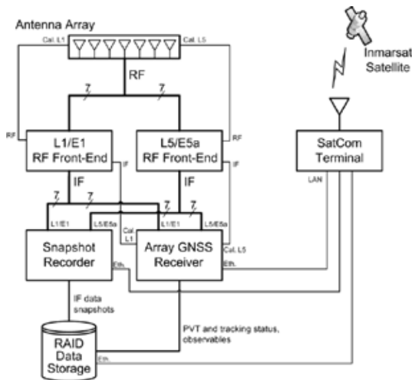
Abb. 2 Blockschriftbild der DLR Messaufbau
