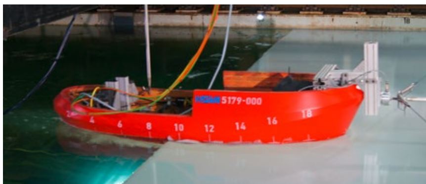
Abb. 18: Modell-Schleppschiff bei der Fahrt in die Eisdecke.
