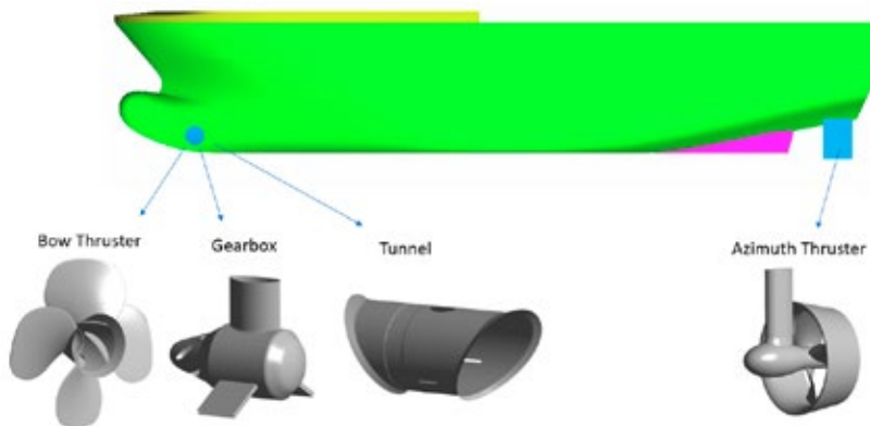
Abb. 6: Untersuchtes Offshore-Versorger-Schiff inklusive Querstrahler und Hauptantrieb.
