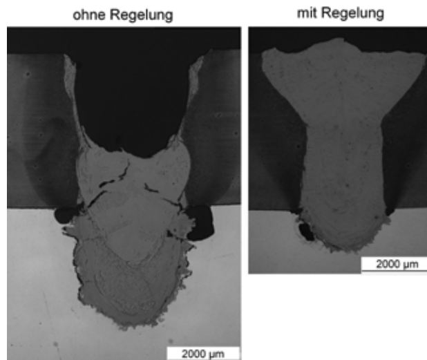
Abb. 11: Querschliffe von Mischverbindungen ohne Einschweißtiefenregelung (links) und mit Einschweißtiefenregelung auf Basis der spektralen Prozessemissionen (rechts) bei einer Vorschubgeschwindigkeit von 0,8 m/min
