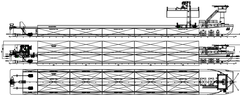
Abb. 4: Entwickeltes WATERTRUCK-Schiffskonzept (mit Bekranung) – Schiffstyp Johann Welker (Klasse IV)
