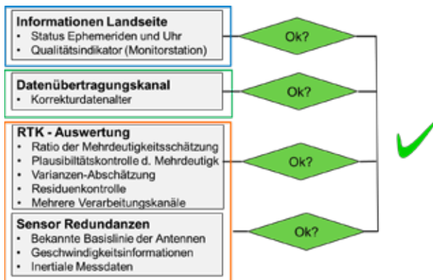
Abb. 7: Integritätskonzept
