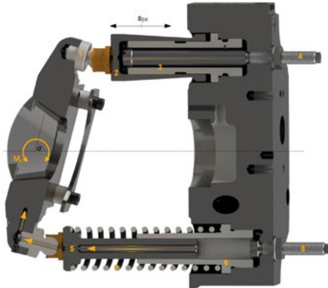
Abb. 6: Finales Stellsystem der Baugröße 4
