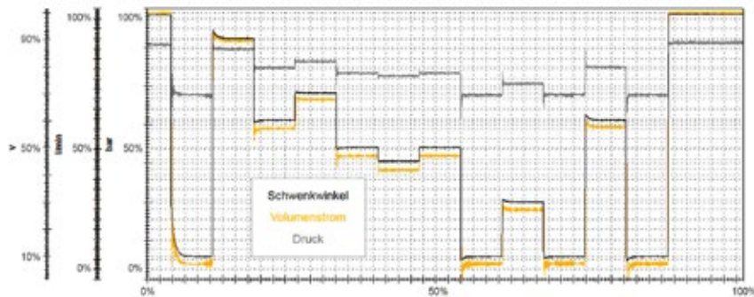
Abb. 11: Definierter Lastzyklus für die Verstellpumpe
