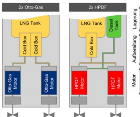
Abb. 1: Zweimotoranlage für den Schiffshauptantrieb mit Otto-Gas Motoren (links) und mit HPDF-Motoren (rechts)
