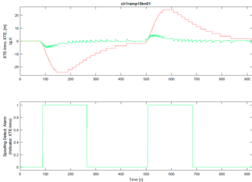
Abb.11: Täuschungsdetektion bei der Bahnregelung
