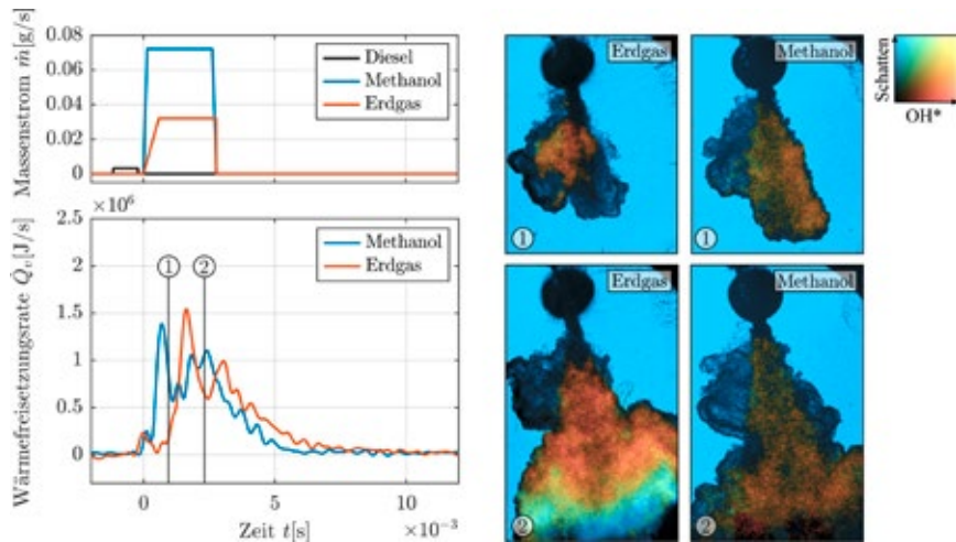
Abb. 5: Ersatz von Erdgas durch Methanol als Hauptbrennstoff: (1) schnellere Entflammung, (2) keine Rußbildung
