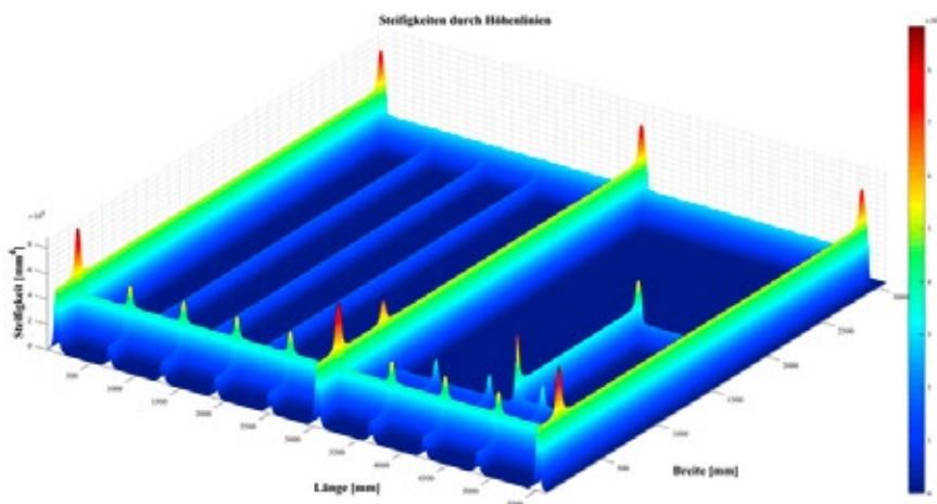
Abbildung 11: Analyse der Steifigkeit am Gesamtdemonstrator (Quelle: Fraunhofer IAPT)
