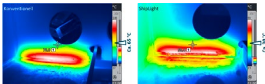
Abb. 14: Beispielhafter Vergleich der Wärmeeinbringung: konventioneller MAG-Prozess und neuer laserunterstützter MAG-Prozess (ShipLight-Prozess) (Quelle: MEYER WERFT)
