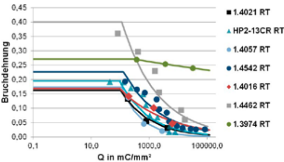
Abb. 31: Zusammenfassende Darstellung der Bruchdehnungen in Abhängigkeit der kathodischen Wasserstoffladung Q für die untersuchten Stähle für Raumtemperatur
