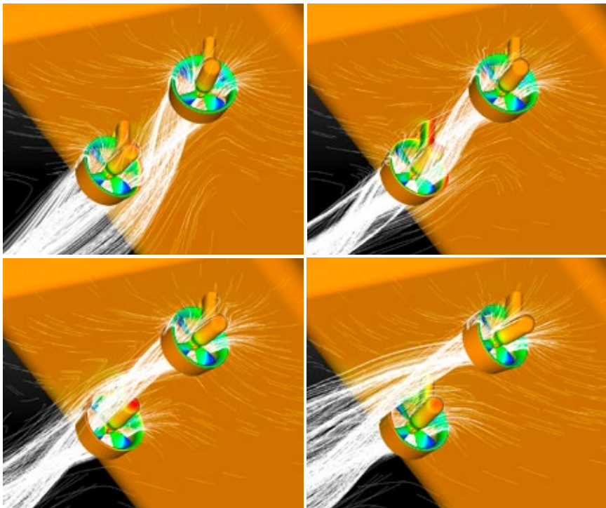
Abb. 1: Variation des Azimuthwinkels des stromaufwärts liegenden Propellers
