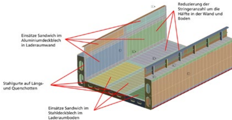
Abb. 5: Leichtbaumaßnahmen zur Gewichtsreduzierung des WATERTRUCK-Schiffsrumfs
