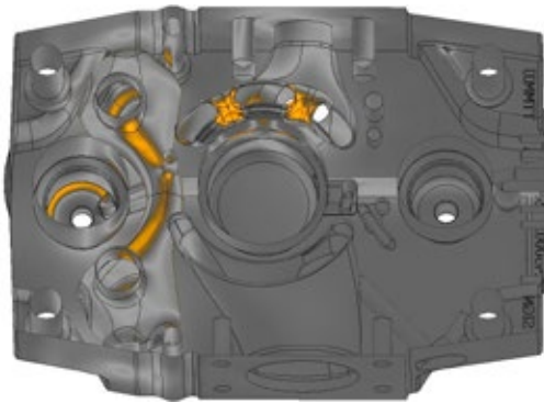
Abb. 8: FEM-Analyse der Anschlussplatte
