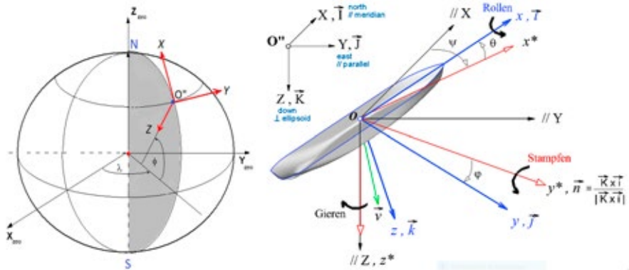
Abbildung 5: Geozentrisches, lokales und schiffsfestes Koordinatensystem
