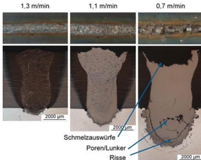
Abb. 4: Aufnahmen von Schweißnahtoberseiten und Querschliffen laserstrahlgeschweißter Mischverbindungen aus dem maritimen Bereich unter Variation der Vorschubgeschwindigkeit
