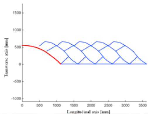
Abb. 3: Beispiel für ein generiertes Bruchmuster eines eisbrechenden Schiffmodells.
