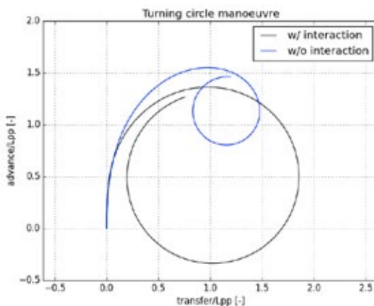
Abb. 9: Berechnetes Drehkreismanöver mit und ohne Berücksichtigung der Wechselwirkung zwischen Propellerstrahl und Rumpf
