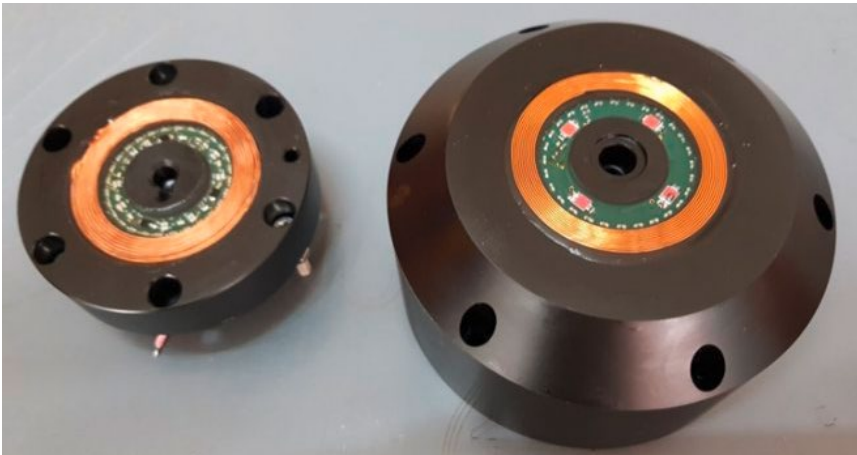
Abb. 15: Rotierende Schnittstelle (kabellose Telemetrie und Energieversorgung).
