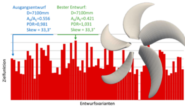
Abb. 9: Ergebnis der Optimierung der Propulsionseffizienz eines Eisklasse Propellers mit einem Panelverfahren.
