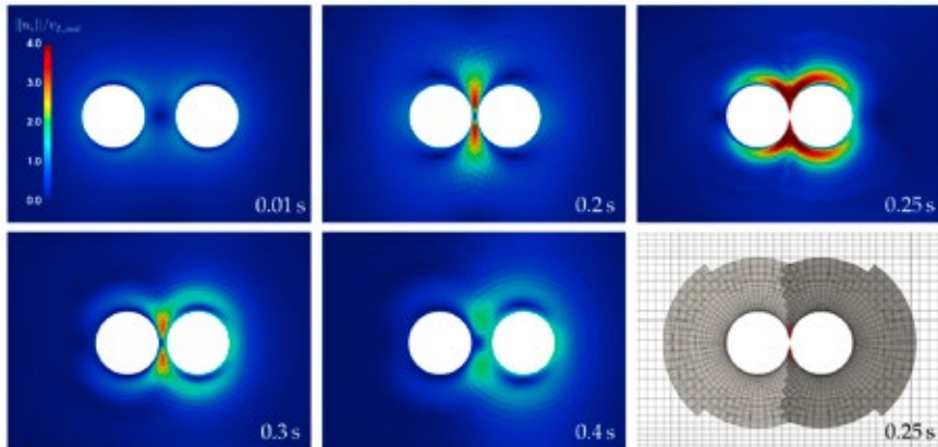
Abb 9: Kollision zweier Zylinder. Unten rechts sind die drei überlappenden Gitter zum Kollisionszeitpunkt dargestellt. Die mit künstlicher Randbedingung behandelten Zellen sind rot markiert.
