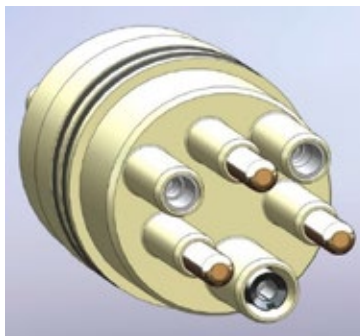
Abb. 27: Iso-Dose
