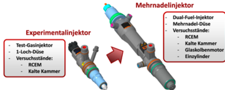
Abb. 7: Gegenüberstellung der HD-Gas-Injektoren
